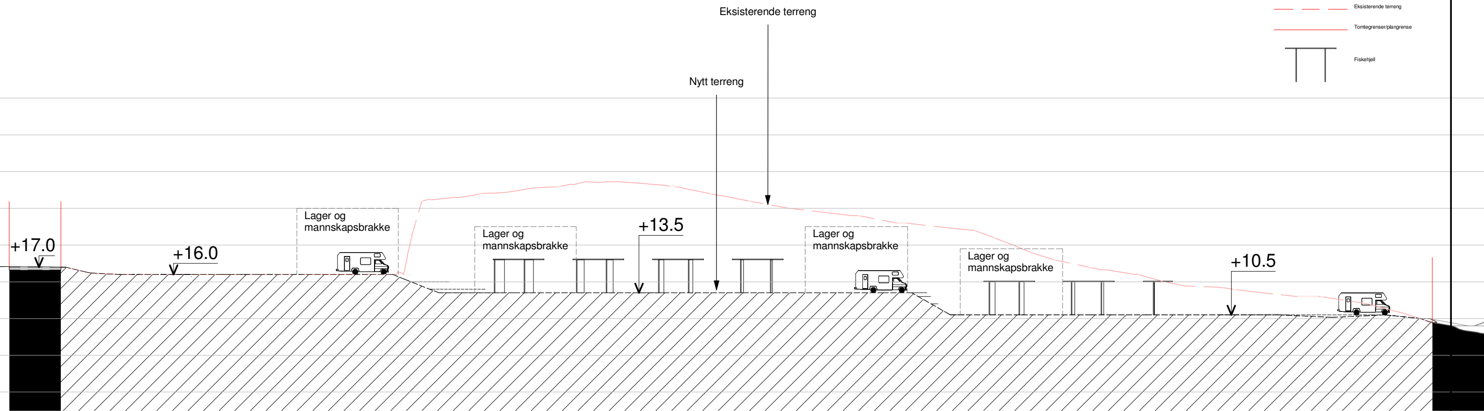
Section 2 1 500 1 : 500
