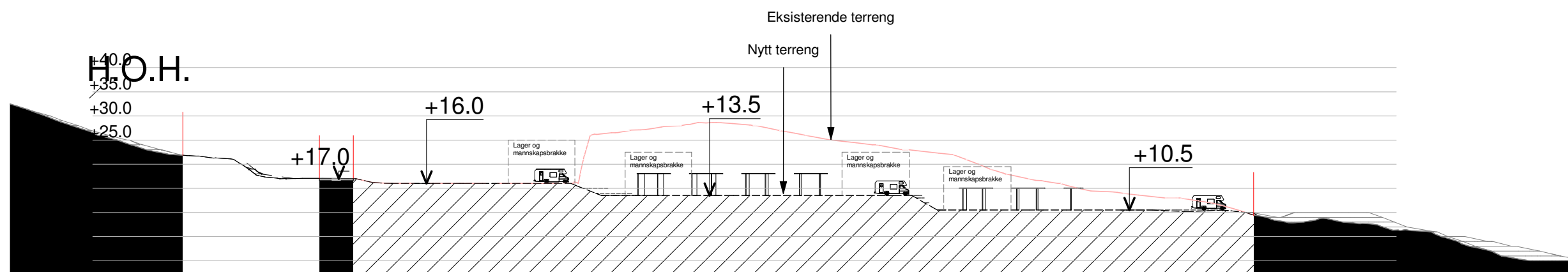
Section 2 1 1000 1 : 1000
