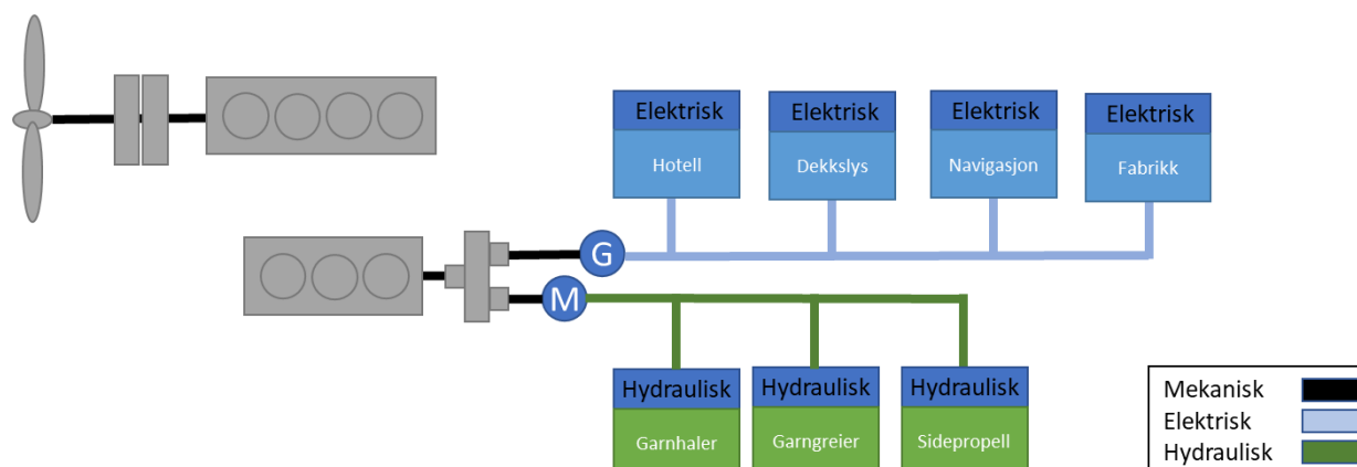
Figur 7: Motorarrangement for større tradisjonell kystbåt - fremdrift fra hovedmotor og elektrisitet og hydraulikk drevet av hjelpemotor. Noen motorarrangement har elektrisk hydraulikkpumpe som dermed drives av det elektriske nettet fra hjelpemotoren.
