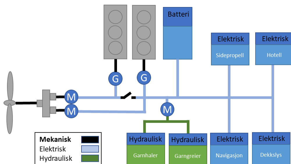
Figur 8: Motorarrangement for større kystfartøy med batterihybrid fremdrift og elektrisk kraftdistribusjon
