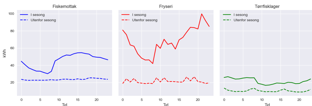
Figur 34 Gjennomsnittlig effektprofil over døgnet i sesong (hel linje) og utenfor sesong (stiplet linje).
