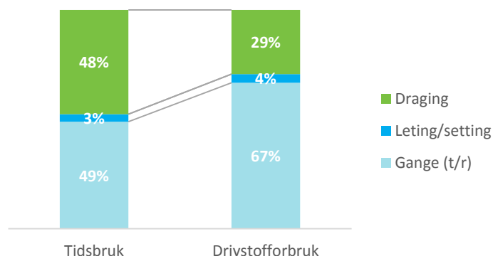
Figur 15 Andel tids- og drivstofforbruk i ulike driftstilstander for et 19m kystfiskefartøy (550hp/410kW) under blåveitefiske på Tromsøflaket. Drivstofforbruket (liter) er estimert basert på informasjon fra fartøyeier om medgått tid og drivstofforbruk (l/t) per driftstilstand.
